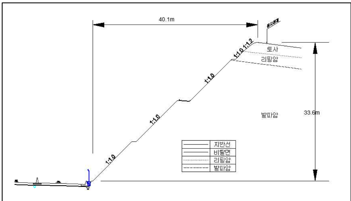
【대표단면 Sta.5+080(영천)】
