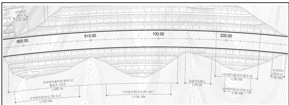
【Sta.4+860~5+300】
