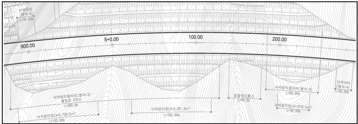
【Sta.4+860~5+300 평면】
