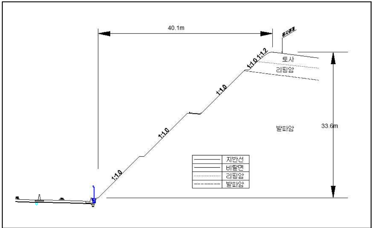
【대표단면 Sta.5+080(영천)】
